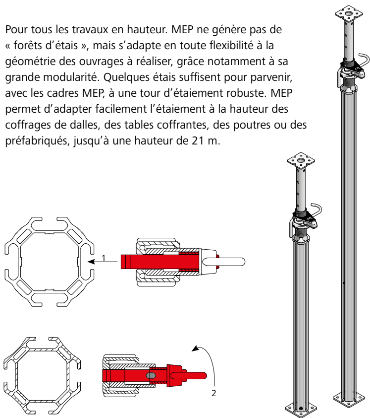
Système de verrouillage rapide du cadre MEP
