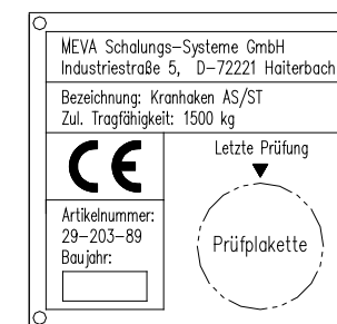
Fig. 7c AluStar / StarTec
