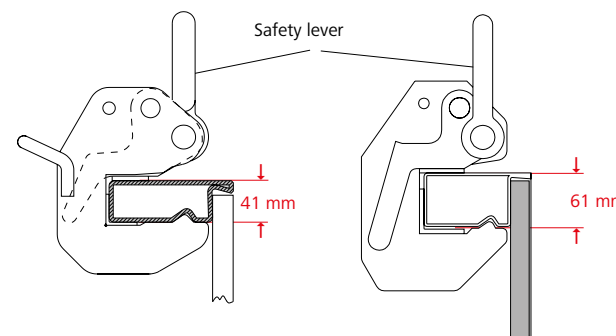
Fig. 1c AluStar / StarTec
