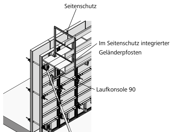
Abb. 20.5 Seitenschutz
