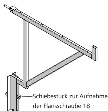
Abb. 20.1 Laufkonsole 90
